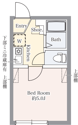
B 1K /15.01 m 2
