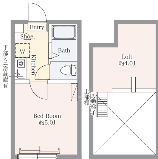
C1 1K+Loft / (15.01 m 2 + Loft 6.61 m 2 ) 生活有効面積 21.62 m 2
