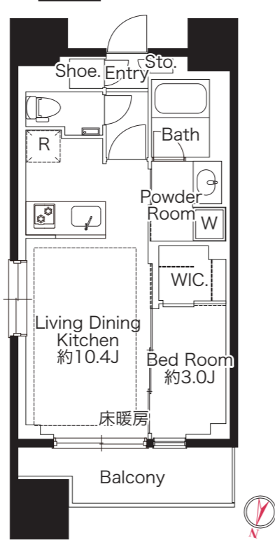
B type 1LDK 35.60㎡
